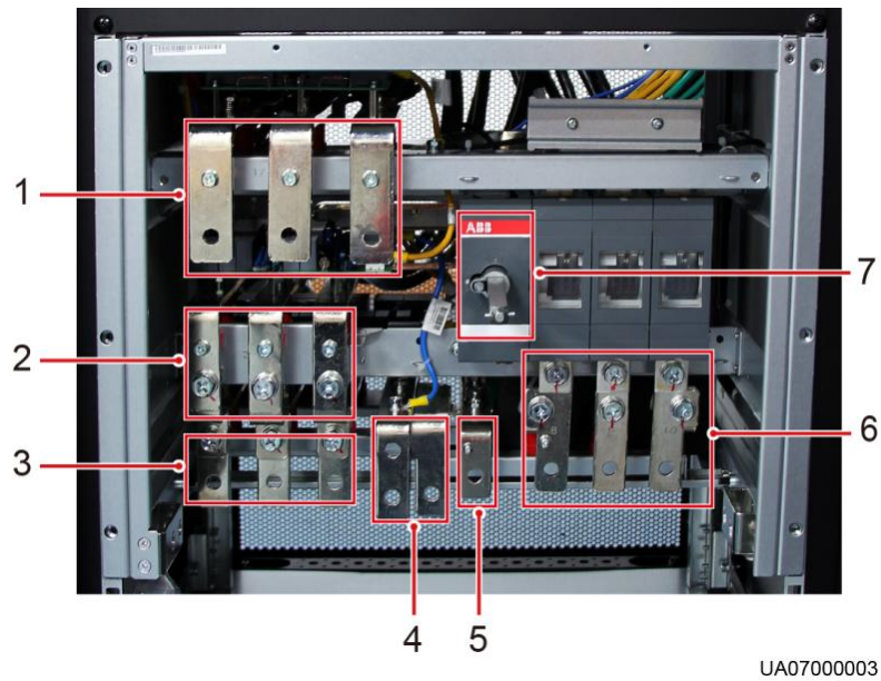
图4-9 配电模块示意图
