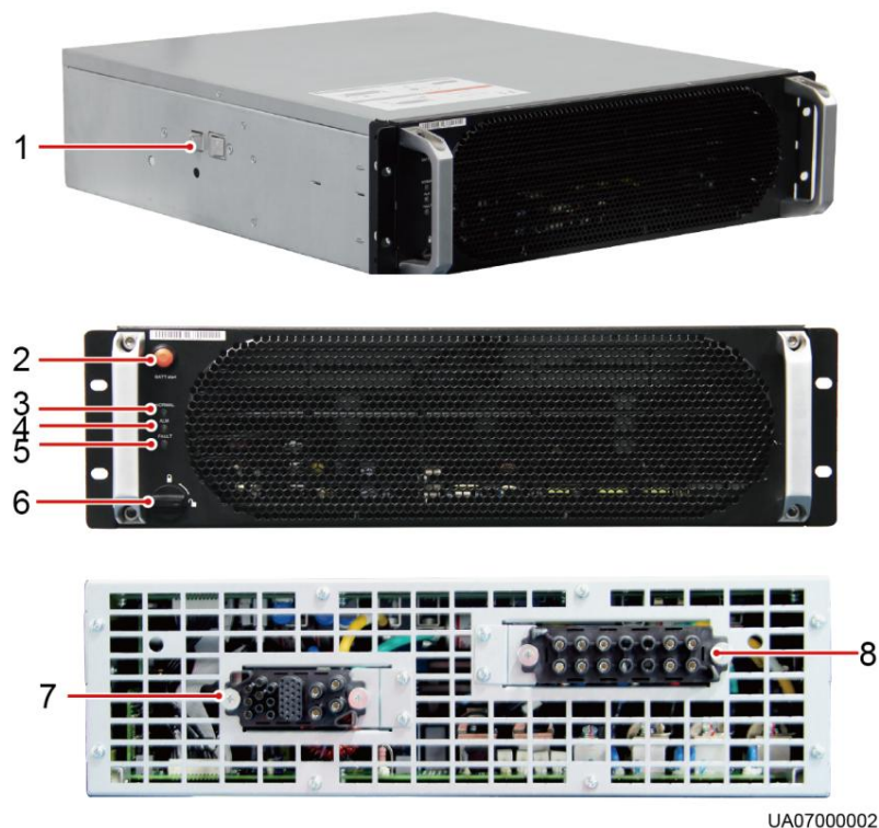
图4-7 旁路模块外观示意图
