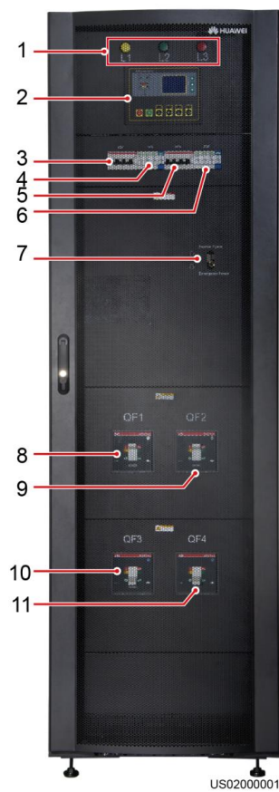
图5-1 配电柜前视图
