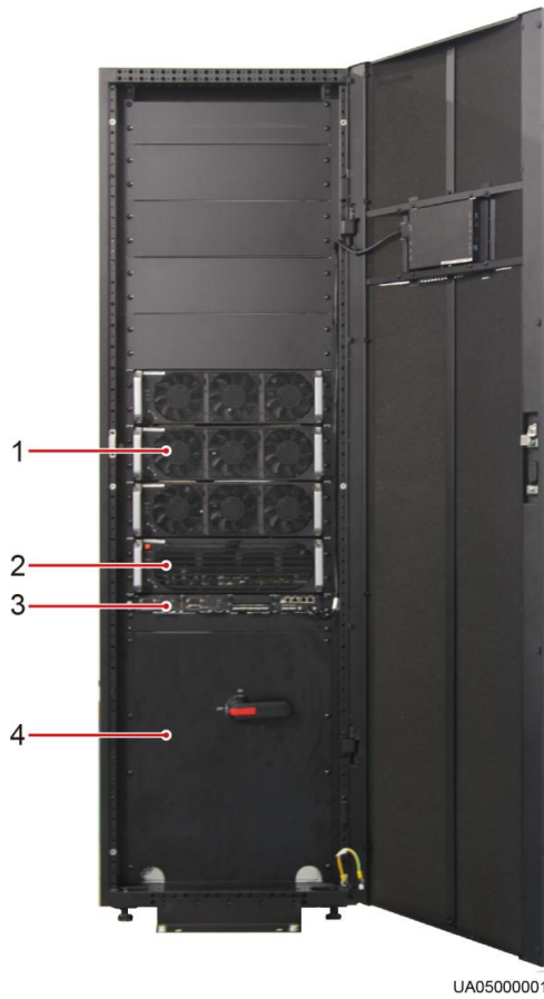
图4-2 UPS5000-E-120K-F120 内部结构
