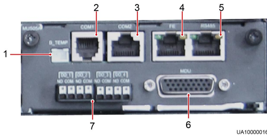
图4-17 监控接口卡面板示意图
