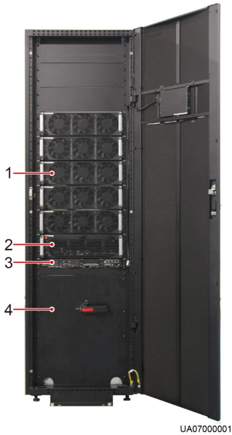
图4-3 UPS5000-E-200K-F200 内部结构
