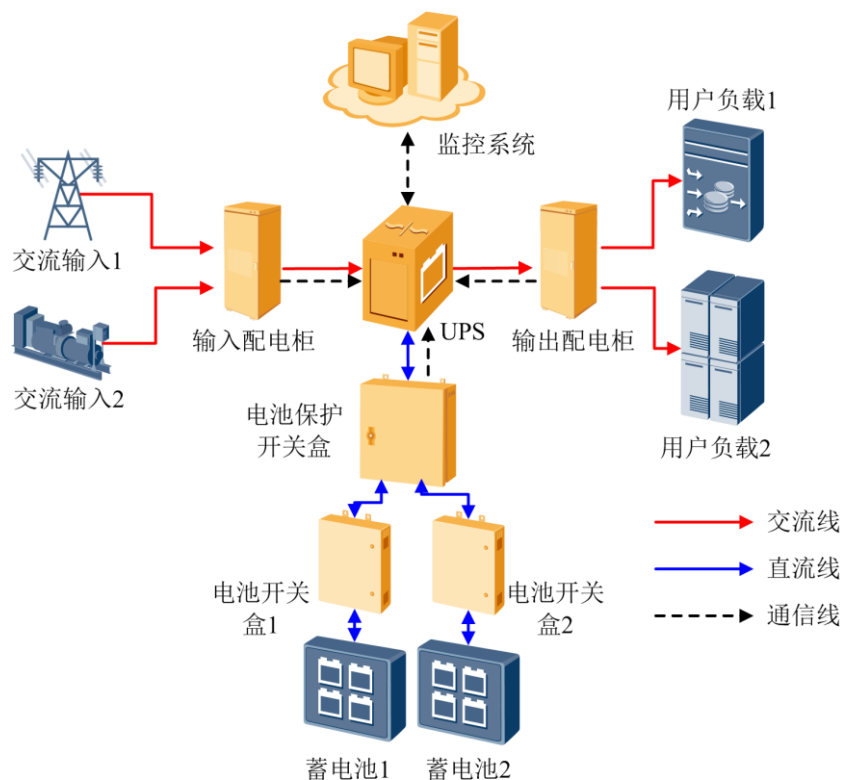
图3-1 UPS5000-E 单机典型应用场景
