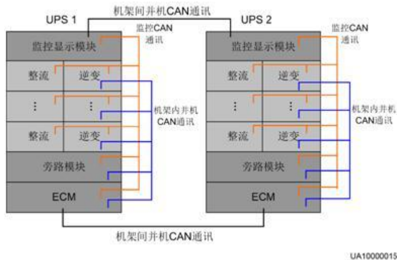
图4-15 CAN 通讯逻辑示意图
