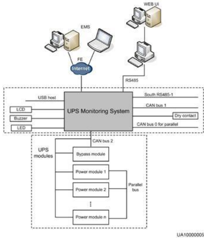
图4-13 监控单元系统在 UPS 系统中的示意图
