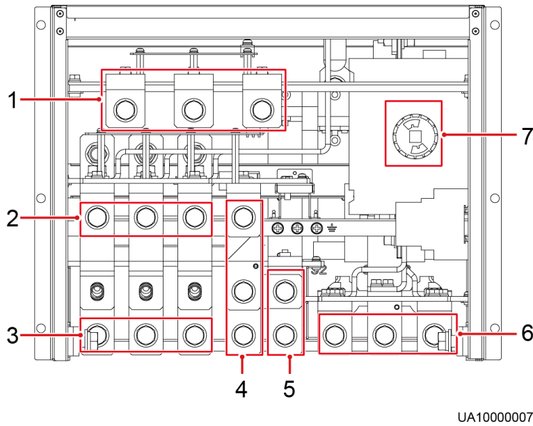
图4-10 配电模块示意图
