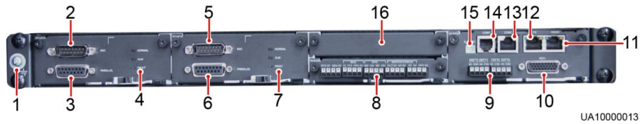
图4-12 控制模块各接口示意图
