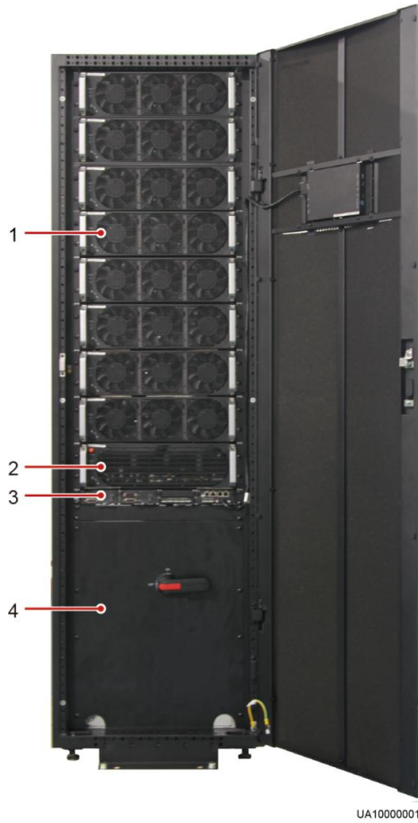
图4-4 UPS5000-E-320K-F320 内部结构
