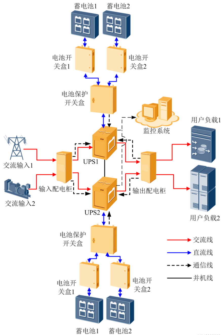
图3-2 UPS5000-E 并机典型应用场景
