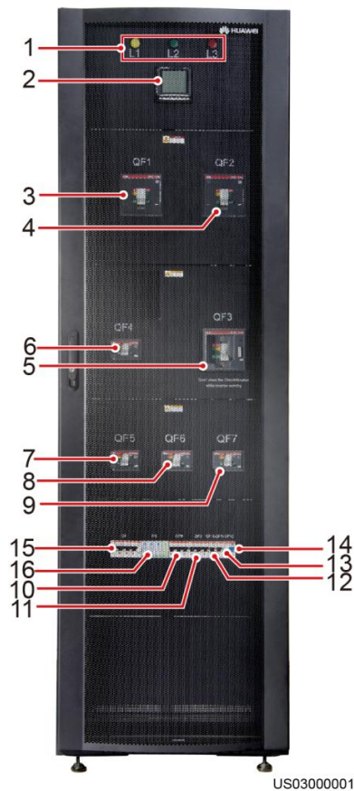
图5-2 配电柜前视图
