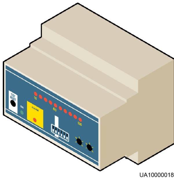
图5-3 电池接地故障仪外观示意图
